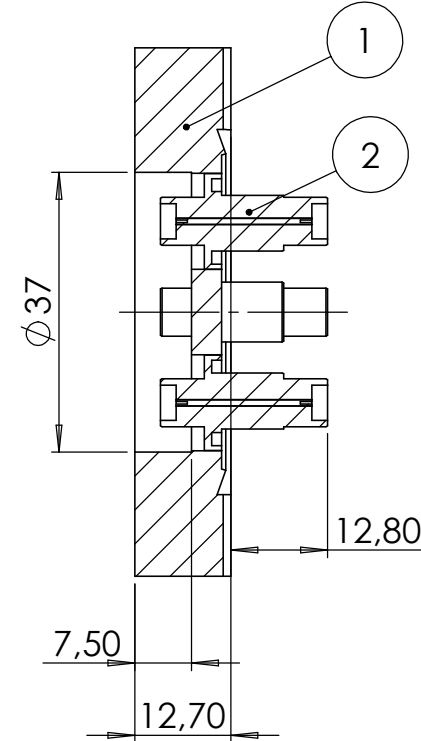
SCHNITT A-A
