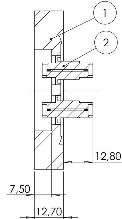
SCHNITT A-A
