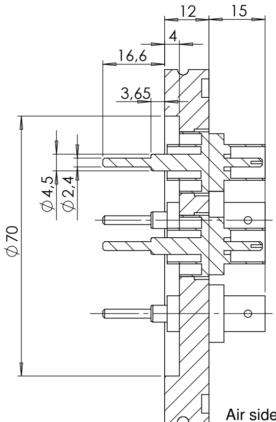
SCHNITT A-A
