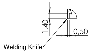
DETAIL A MAßSTAB 2 : 1
