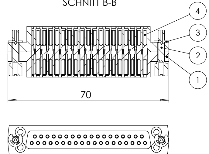
SCHNITT B-B
